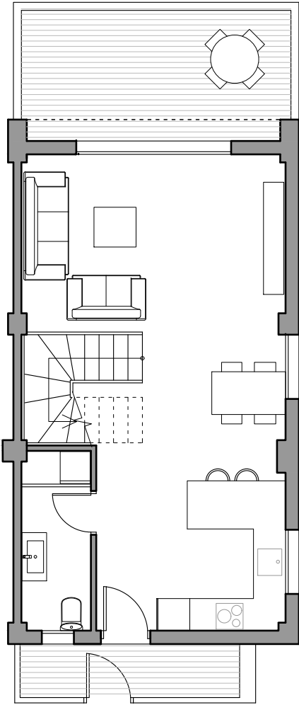
PLANTA BAJA
